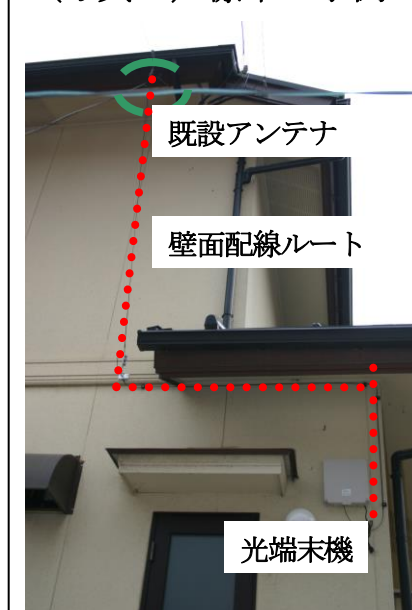
（写真2）標準工事例
